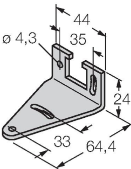
Montážní úhelník, nerez, pro závitová pouzdra M30
