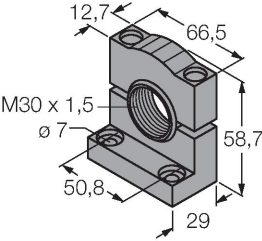
Montážní úhelník úhlový, nerez, pro senzory se závitem M30, otvory pro nastavení směru
