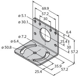
Montážní úhelník úhlový, nerez, pro senzory se závitem M30, otvory pro nastavení směru
