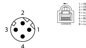
Schéma zapojení
