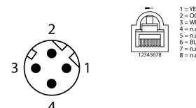
Schéma zapojení
