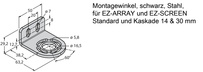
EZA-MBK-11 3071470
