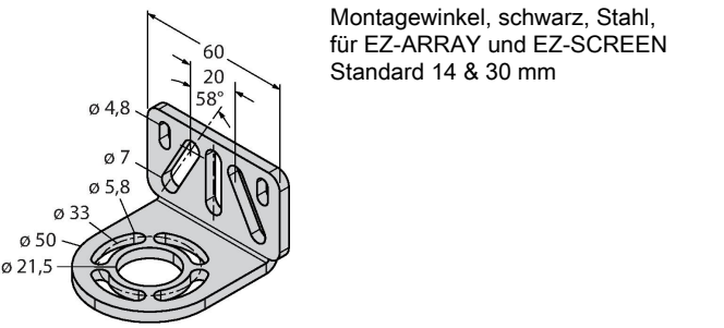
EZA-MBK-20 3072587
