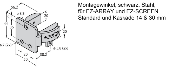
EZA-MBK-12 3071756
