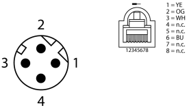
Schaltplan
