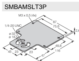
3073132 panel de montaje, acero inoxidable, para modelo LT3
