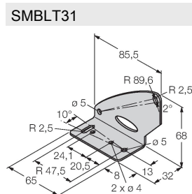
3068505 ángulo de montaje, acero inoxidable, para modelo LT3
