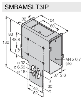
3073442 carcasa de protección con cristal protector, acero inoxidable, para modelo LT3
