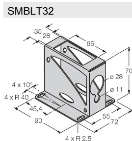
3069236 carcasa de protección, acero inoxidable, para modelo LT3
