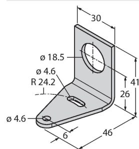
SMBQS18AF
