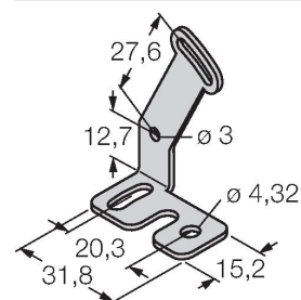
SMBQS18AF
