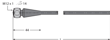
Dibujo acotado Tipo N.º de ID RKH4.5-2/TFG 6933455
