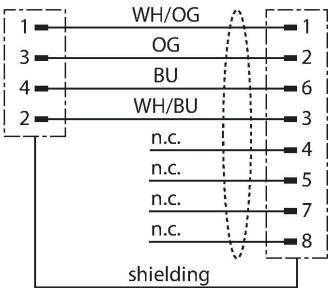
diagrama de conexiones
