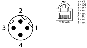
schéma de connexions
