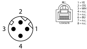
schéma de connexions
