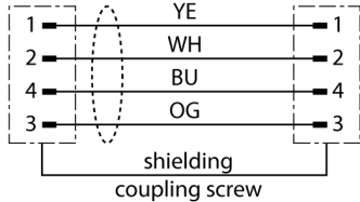
schéma de connexions
