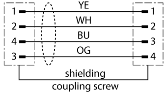
schéma de connexions
