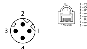
schemat obwodu
