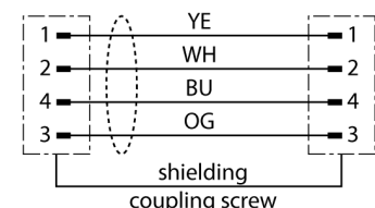
schemat obwodu
