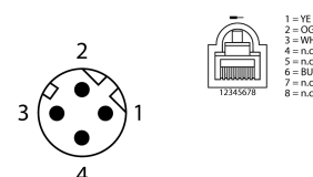
Schema de conexiuni
