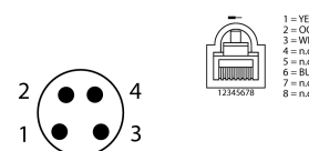
Schema de conexiuni
