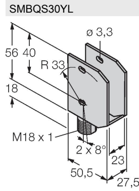
SMBQS30YL 3072741 Güvenlik camı paneli bulunan koruyucu gövde, paslanmaz çelik, QS30 serisi için
