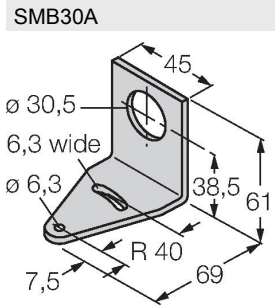
SMB30A 3032723 Montaj braketi, dikdörtgen paslanmaz çelik, 30 mm dişli sensörler için
