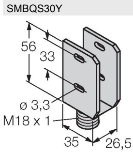
SMBQS30Y 3002811 Koruyucu gövde, paslanmaz çelik, QS30 serisi için
