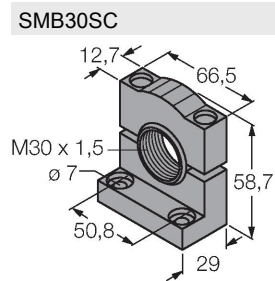
SMB30SC 3052521 Montaj braketi, PBT siyah, 30 mm dişli sensörler için, döndürülebilir
