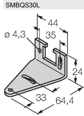
SMBQS30L 3002809 Montaj braketi, paslanmaz çelik, QS30 serisi için
