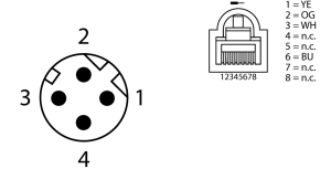
Devre şeması
